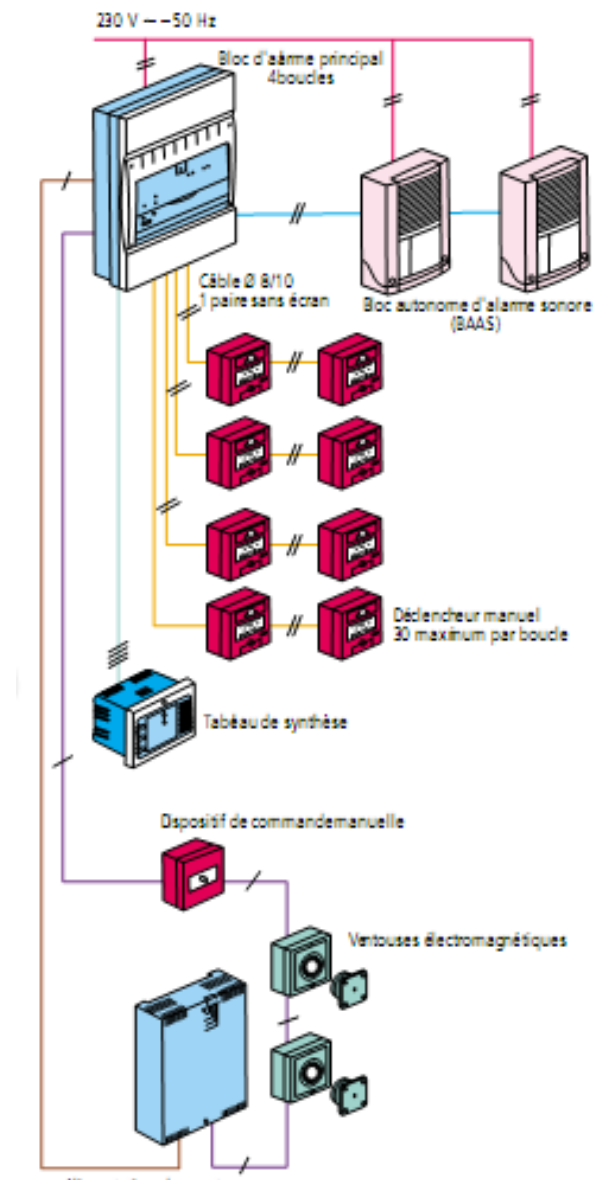
Schéma de principe d'installation (d'après Legrand).
